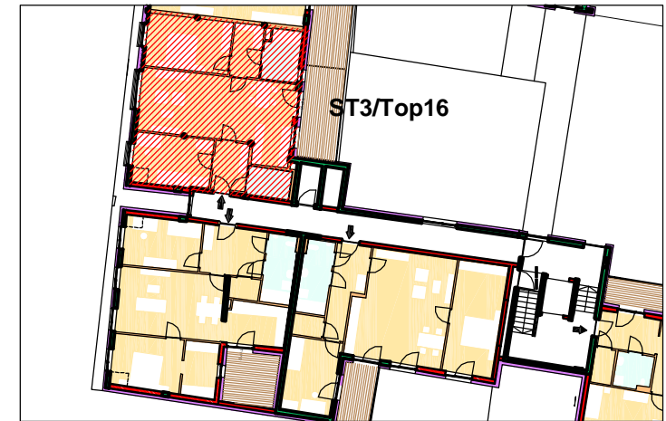
LAGESITUATION
